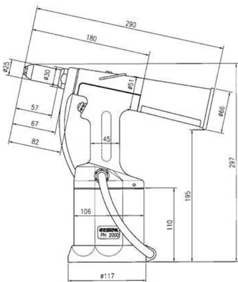
Dimensões em mm
